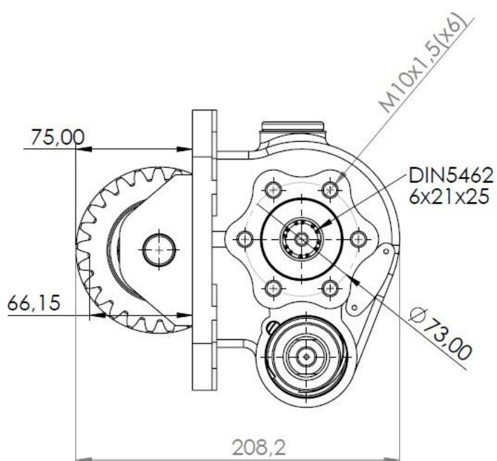
Модель коробки передач HINO LJ 06 S
