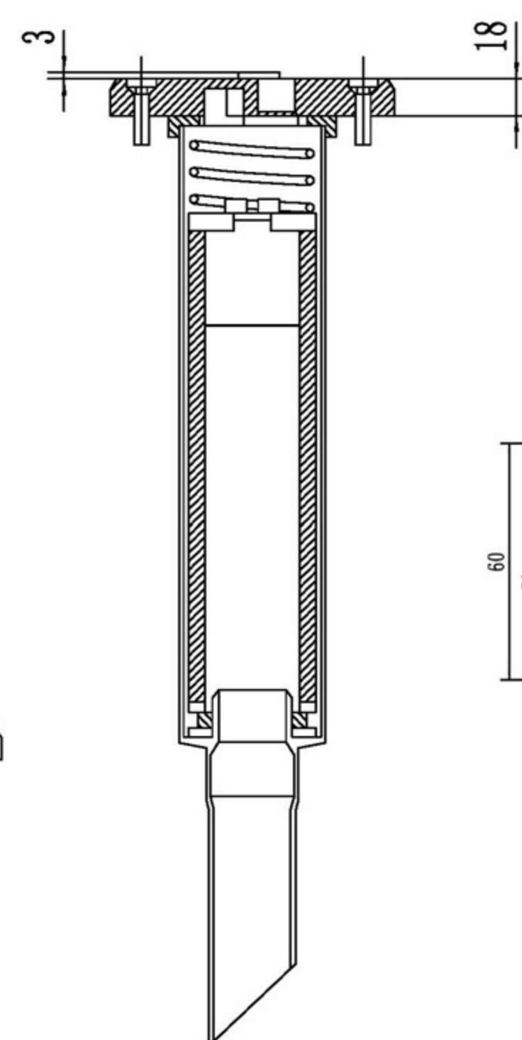
Масляный фильтр
