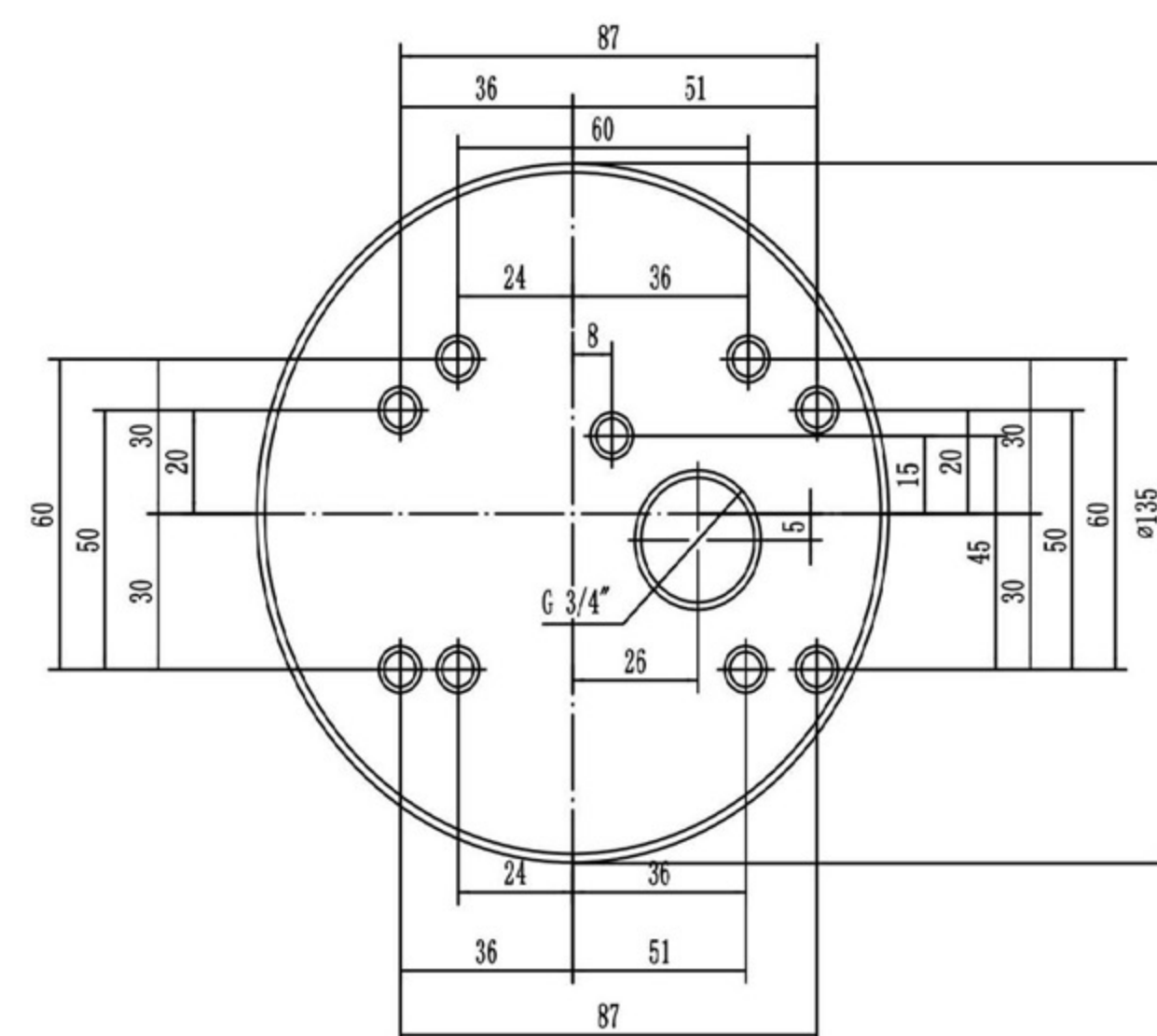
Плита для распределителя
